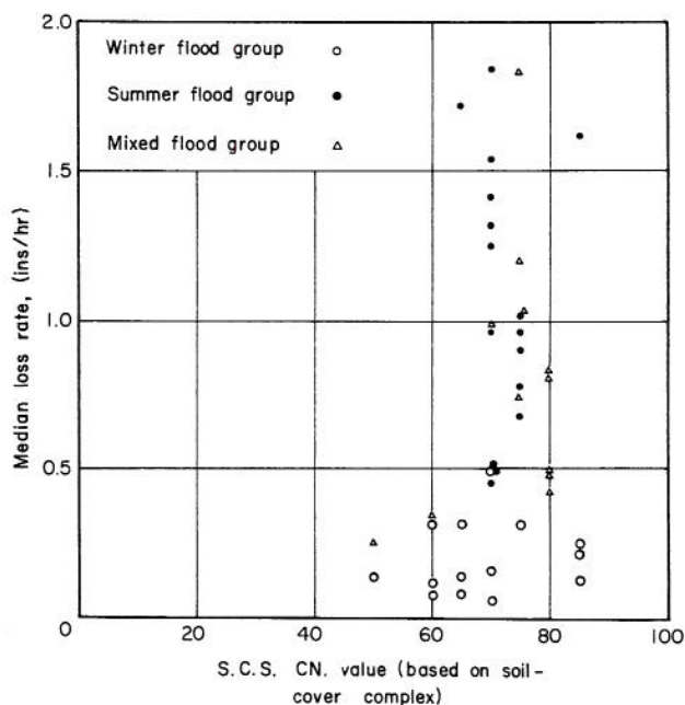
Fig. 19 S. C. S. CN versus median loss rate
